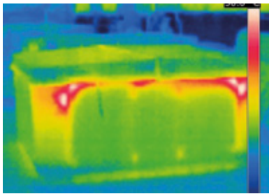
Test di dispersione termica effettuato con il sistema EcoSpa
