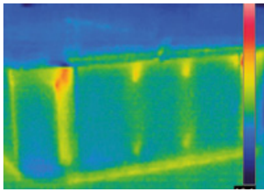
Verifica di perdita di calore con sistema Nordic Insulation System
